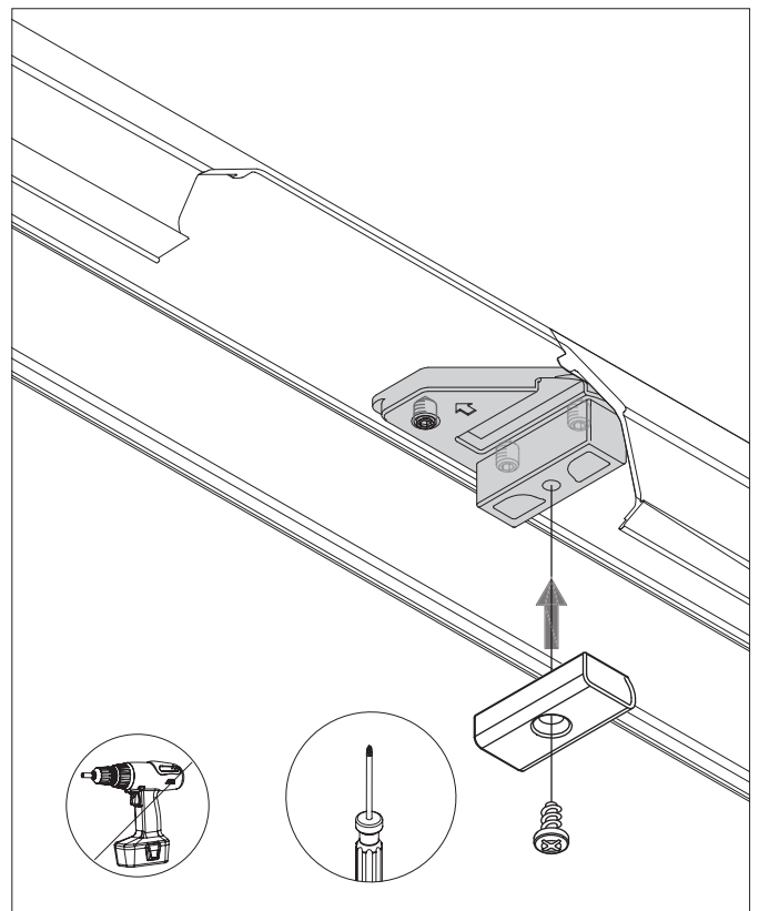
8. Ruuvaa ohjaimen korotuspala paikoilleen. Huomioi oikea asento.
